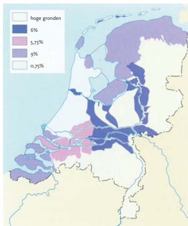
Figuur 6. Kans van overstroming in een mensenleven, gebaseerd op de wettelijke overschrijdingsfrequenties en een gemiddelde levensduur van 75 jaar [bron: 158].
